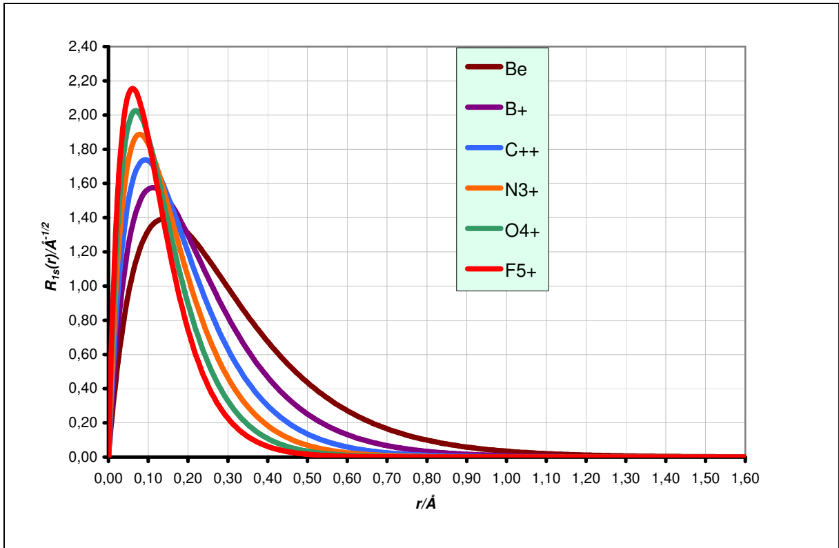
graf 10 : 1s valne funkcije za ione Be, B + , C ++ , N 3+ , O 4+ , F 5+ sa 4 elektrone u HFA
