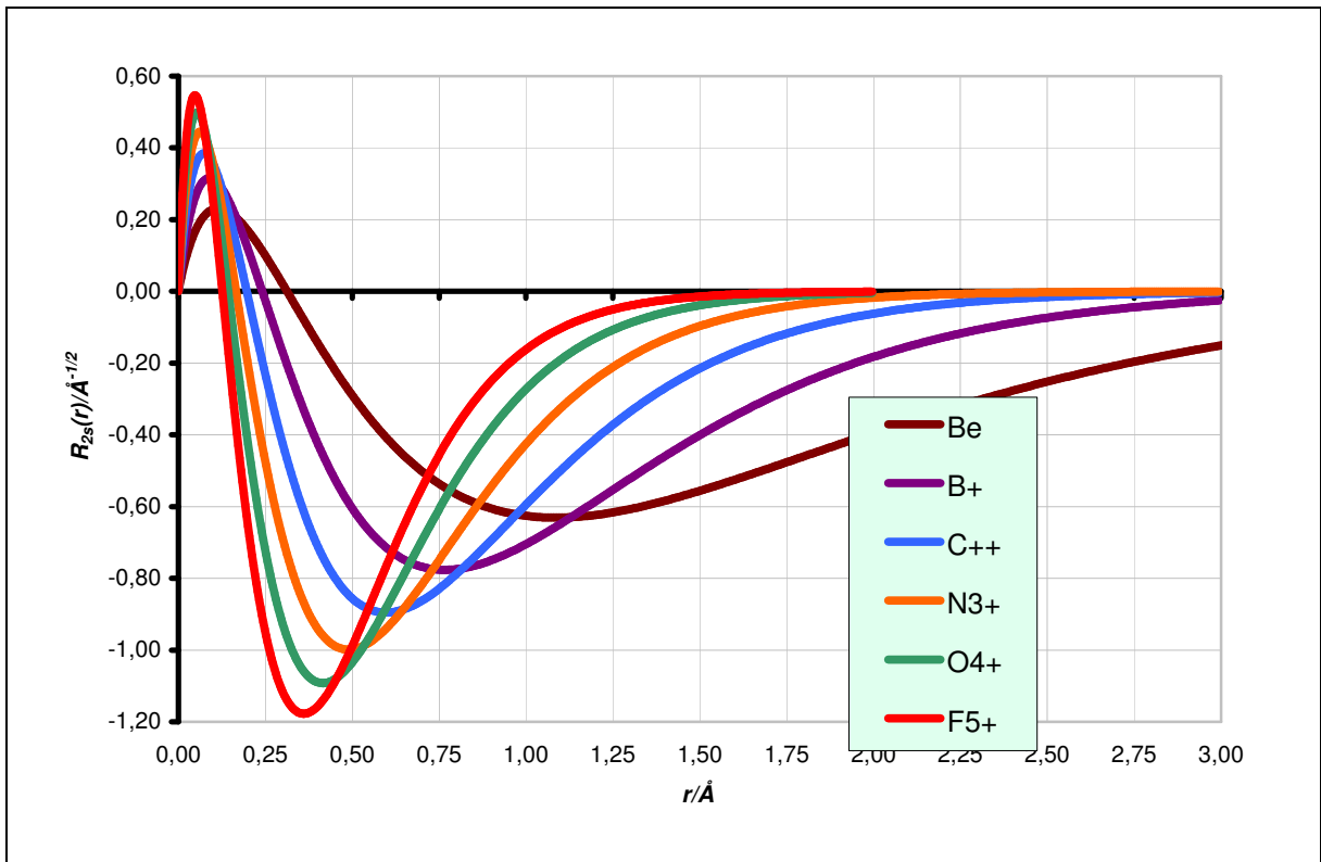
graf 11 : 2s valne funkcije za ione Be, B + , C ++ , N 3+ , O 4+ , F 5+ sa 4 elektrone u HFA
