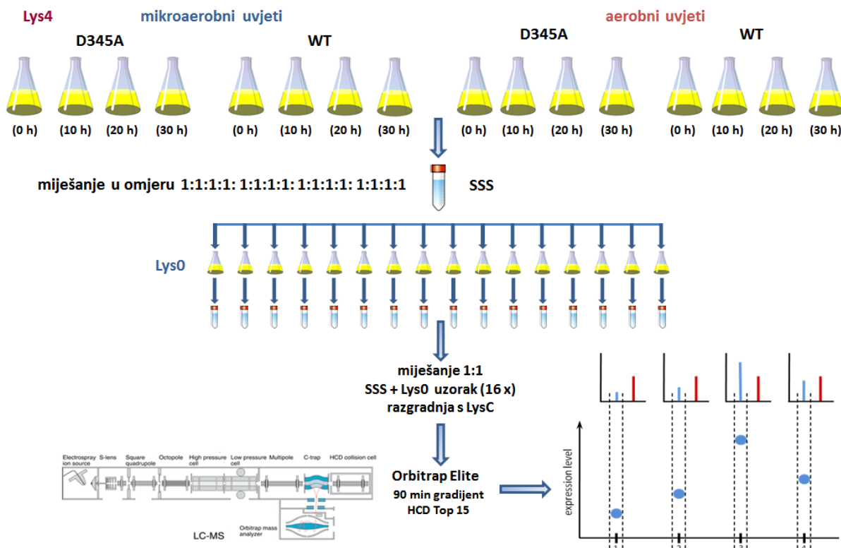
Slika 4.25 Shema postave eksperimenta SuperSILAC. Lys4- “teški” lizin, Lys0 –“laki” lizin, SSS – SuperSILAC standard, D345A – soj E. coli D345A LeuRS MG1655, WT – soj E. coli WT LeuRS MG1655.
