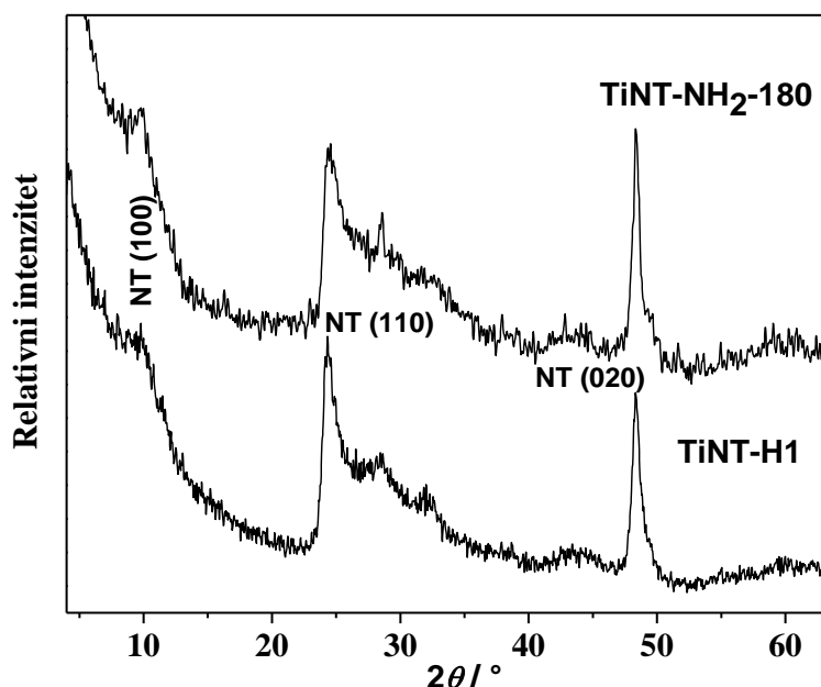
Slika 58. Rendgenski difraktogrami na sobnoj temperature prije grijanja za protonirani oblik nanocjevčica (TiNT-H1) i za TiNT-NH 2 -180 nanocjevčice modificirane APTMS-om 181 .
