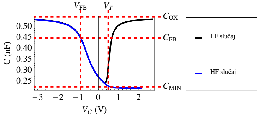
Slika 1.28: Simulacija LF i HF C-V karakteristika MOS strukture s parametrima d_{\text{OX}} = 200 \text{ nm} , N_A = 1 \cdot 10^{15} \text{ cm}^{-3} , V_{fb} = 0.88 \text{ V} na površini kontakta A = 0.001^2 \pi [m^2] .
