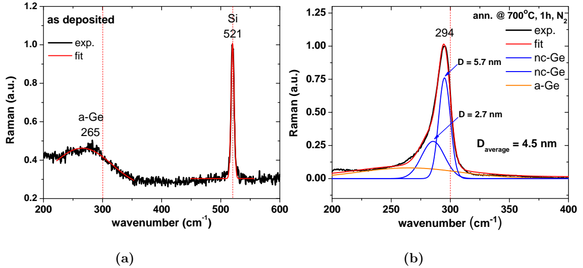
Slika 3.2: Raman spektar: (a) tek napravljenog (as-dep.) uzorka u kojem je jedan sloj Ge-obogaćenog oksida i prilagoda mjerenja na signal a-Ge i kristalinične podloge Si, (b) područje signala a-Ge nakon grijanja 1h na 700°C i prilagodbe na signale a-Ge i nanokristaliničnog Ge.
