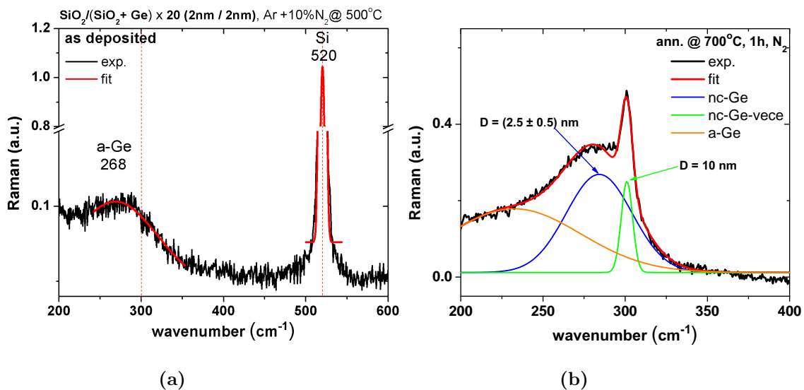
Slika 3.4: Raman spektar: (a) tek napravljenog (as-dep.) uzorka napravljenog naizmjenično s 20 slojeva Ge-obogaćenog \text{SiO}_2 i \text{SiO}_2 svaki debljine 2 nm i prilagoda spektra na amorfni Ge (a-Ge) i kristaliničnu podlogu Si, (b) područje signala a-Ge nakon grijanja 1h na 700^\circ\text{C} u atmosferi \text{N}_2 i prilagodba na signale amorfno Ge (a-Ge), većih nanočestica Ge (nc-Ge-veci) i nanočestica Ge (nc-Ge).
