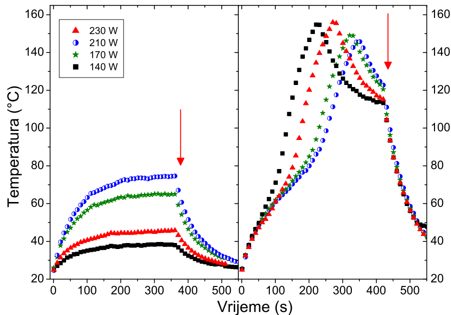
Slika 5.27: Temperatura cijevi prilikom procesa napanavanja u CH 4 plazmi (lijevo) i uklanjanja slojeva O 2 plazmom (desno). Napanavanje je uvijek bilo s 25 Pa CH 4 , a uklanjanje s 33 Pa O 2 i 220 W. Crvene strelice označavaju isključivanje plazme.
