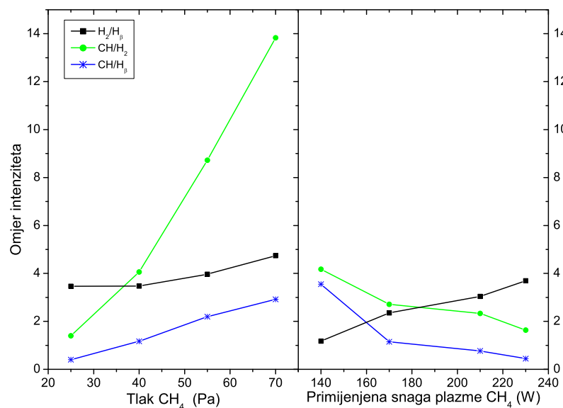
Slika 5.23: Ovisnost omjera intenziteta molekulske vrpce CH (A-X), atomske linije H β i Q1 linije iz (0,0) Fulcherove vrpce (na 602 nm) o tlaku (fiksna snaga od 230 W) (a) i primijenjenoj snazi (fiksni tlak od 25 Pa) (b).
