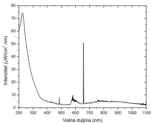
Slika 4.10: Teorijski spektar kalibracijske lampe DH-CAL.
