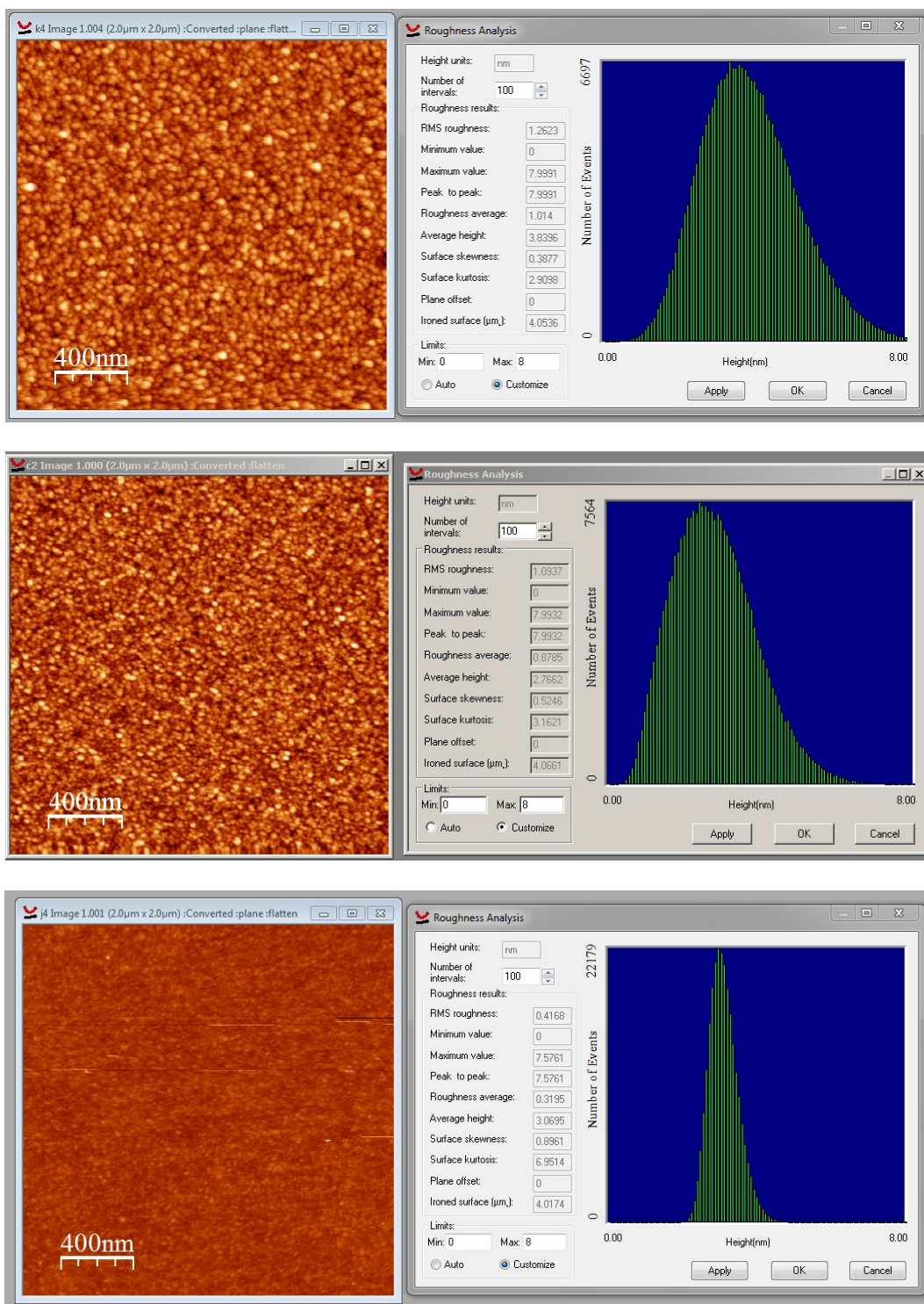
Slika 66. Ovisnost hrapavosti površine o energiji ionskog snopa. Gore: 34 MeV, sredina: 28 MeV, dole: 23 MeV. Primjenjena doza 10^{13} iona/cm 2 , kut ozračavanja 1^0 u odnosu na okomicu. Primjetna je mnogo manja hrapavost i uža distribucija visina za uzorak ozračen s 23 MeV ionima joda.
