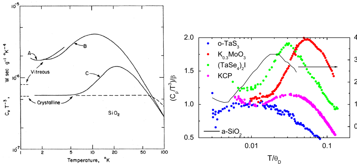
Slika 30 Lijevo: bozonski vršak u kristalnom i amorfnom kvarcu, desno: bozonski vršak u više VGN sistema u usporedbi sa amorfnim kvarcom.
