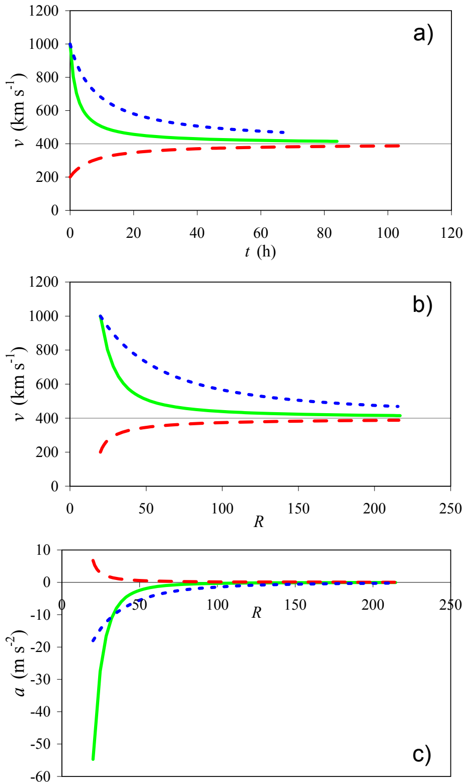
Slika 5.13.: Kinematika izbačaja izračunata s brzinom Sunčevog vjetra od w_c = 400 \text{km/s} (asimptotska siva linija): (a) brzina kao funkcija vremena; (b) brzina kao funkcija udaljenosti; (c) ubrzanje kao funkcija udaljenosti. Crtkana linija opisuje izbačaj s v_0 = 200 \text{km/s} i M = 10^{12} \text{kg} , puna linija s v_0 = 1000 \text{km/s} i M = 10^{12} \text{kg} , dok točkana linija odnosi se na izbačaj s v_0 = 1000 \text{km/s} i M = 4 \times 10^{12} \text{kg} .
