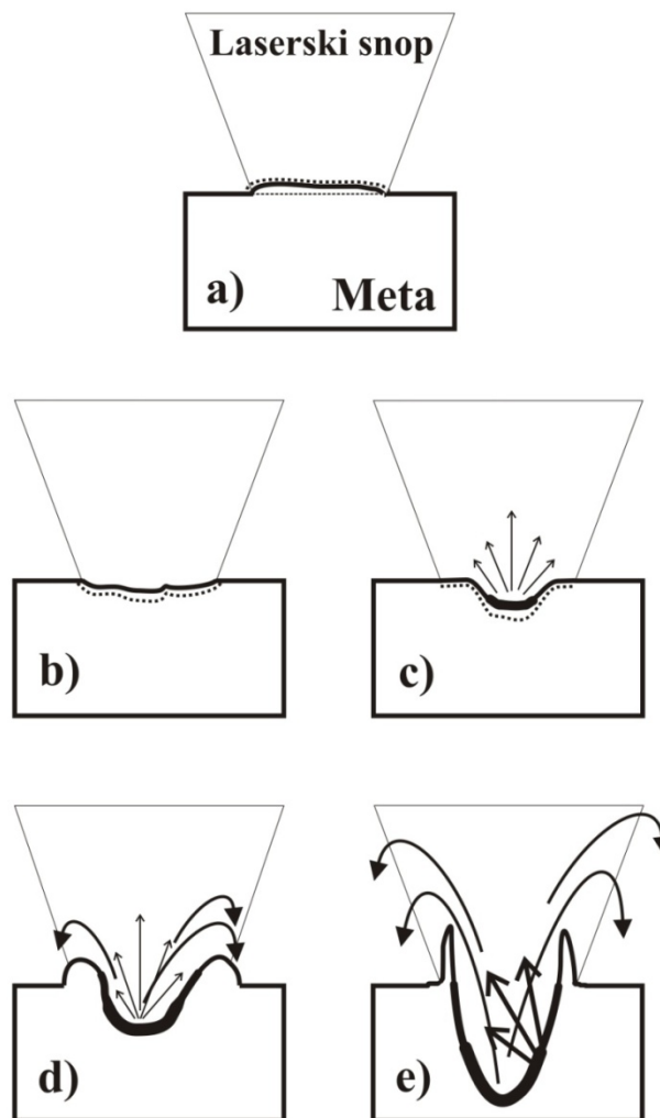
Slika 6.49. Ilustracija raznih faza laserske ablacije ovisno o broju pulseva: a) početak ablacije (nekoliko pulseva) – promjena morfologije, izdizanje površine zahvaćene laserskim pulsem iznad okolne površine, b) početak bušenja mete (do nekoliko desetaka pulseva) – promjena morfologije; zaglađen centar ablacije i koncentrične kružnice smrznutih akustičnih valova okolo, c) početak formiranja kratera (nekoliko desetaka do stotinjak pulseva) – reducirana površina ablacije, d) prolongirana ablacija (do nekoliko stotina pulseva) – formiranje krune, te mikronske kapljice oko kratera i e) ekstenzivna ablacija (nekoliko stotina pulseva i više) – veliki omjer dubine i radijusa kratera, redepozicija ablatiranih čestica na unutarne stjenke kratera, formiranje visoke krune oko kratera, izbačaj mnoštva mikronski kapljica oko kratera, defokusiranje laserskog pulsa.
