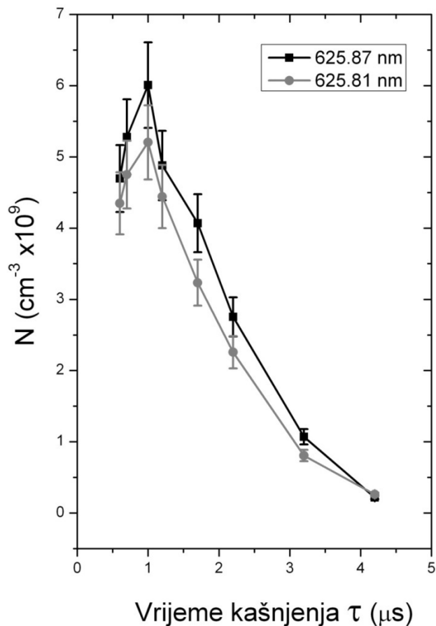
Slika 6.11. Koncentracija ablatiranih atoma titana u stanju {}^3F_{J=3} (sivi kružići) i {}^3F_{J=3} (crni kvadratići) u ovisnosti o vremenu kašnjenja laserskih pulseva za ablaciju \tau . Vremenski prozor bio je T = 200 ns i \Delta T = 200 ns. Spektri su snimljeni na d = 0.5 cm i s = 0.2 cm.
