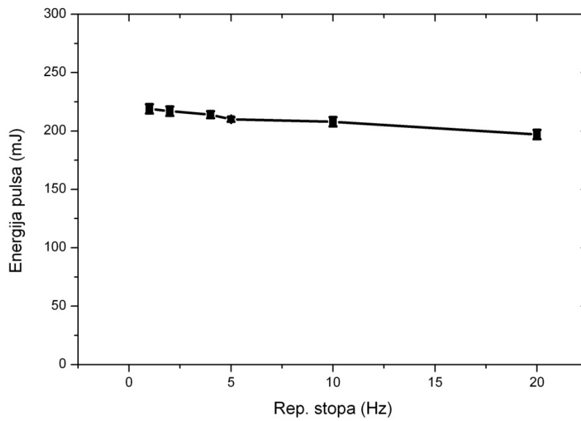
Slika 6.54. Ovisnost energije laserskog pulsa lasera-1 o repeticijskoj stopi.
