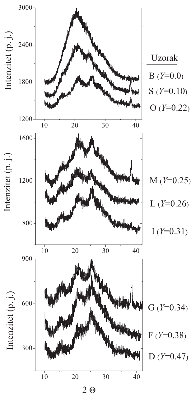
Slika 6.3: Difraktogrami uzoraka PANI-HCl različitih stupnjeva dopiranja. Pomoću difraktograma se može pratiti evolucija rasta Braggovih maksimuma i smanjenja amorfno signala povećanjem stupnja dopiranja, Y . Braggov maksimum koji se pojavljuje na oko 2\theta=40^\circ dolazi od srebrne paste koja je korištena za izradu kontakata kod transportnih mjerenja.
