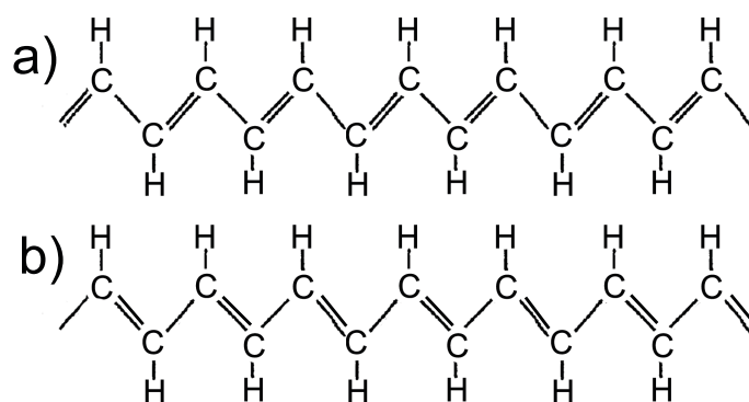
Slika 2.5: Strukturna kemijska formula konformacijskog izomera trans -PA. Strukture a) i b) su ekvivalentne (jednakih energija), stoga je osnovno stanje degenerirano.
