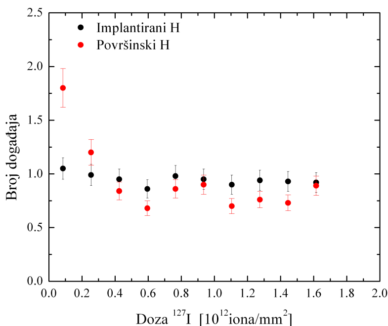
Slika 6.7 Ovisnost stabilnosti površinskog i implantiranog vodika o dozi ulaznog snopa
