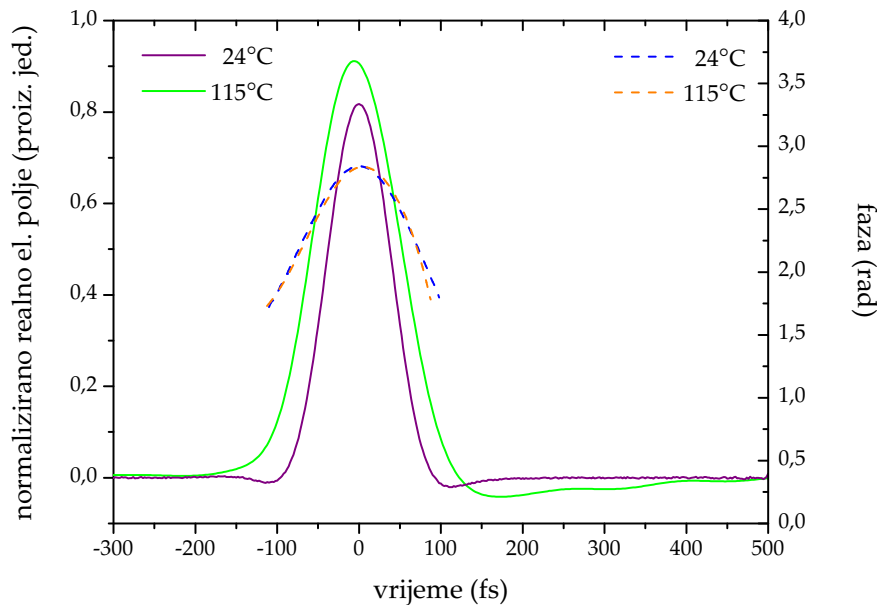
Slika 4.9: Rekonstruirana anvelope električnog polja pulsa iz eksperimentalnih FROG spektrograma za dvije temperature para rubidija. Crtkane linije odnose se na fazu pulsa u području gdje je puls dobro definiran. Oblik faze pulsa upućuje na postojanje linearnog cvrkuta.
