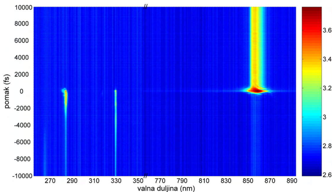
Slika 5.12: Tranzijenti različitih frekventnih komponenti u signalu četverovalnog miješanja snimljeni spektrometrom. Valna duljina femtosekundnih pulseva podešena je na \lambda_c = 854 \text{ nm} . P(\text{He})=25 \text{ Torr} , T_{\text{Na}} = 420^\circ\text{C} ( N_{\text{Na}} = 8.8 \times 10^{15} \text{ cm}^{-3} , N_{\text{Na}_2} = 2.1 \times 10^{14} \text{ cm}^{-3} ). P_{\text{ulaz}} = 5 \mu\text{J} . Zbog isticanja slabijih signala prikazan je logaritam intenziteta.
