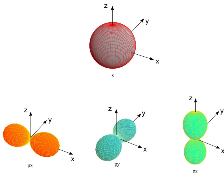
Slika A.1 – 1s i 2p atomske orbitale.
