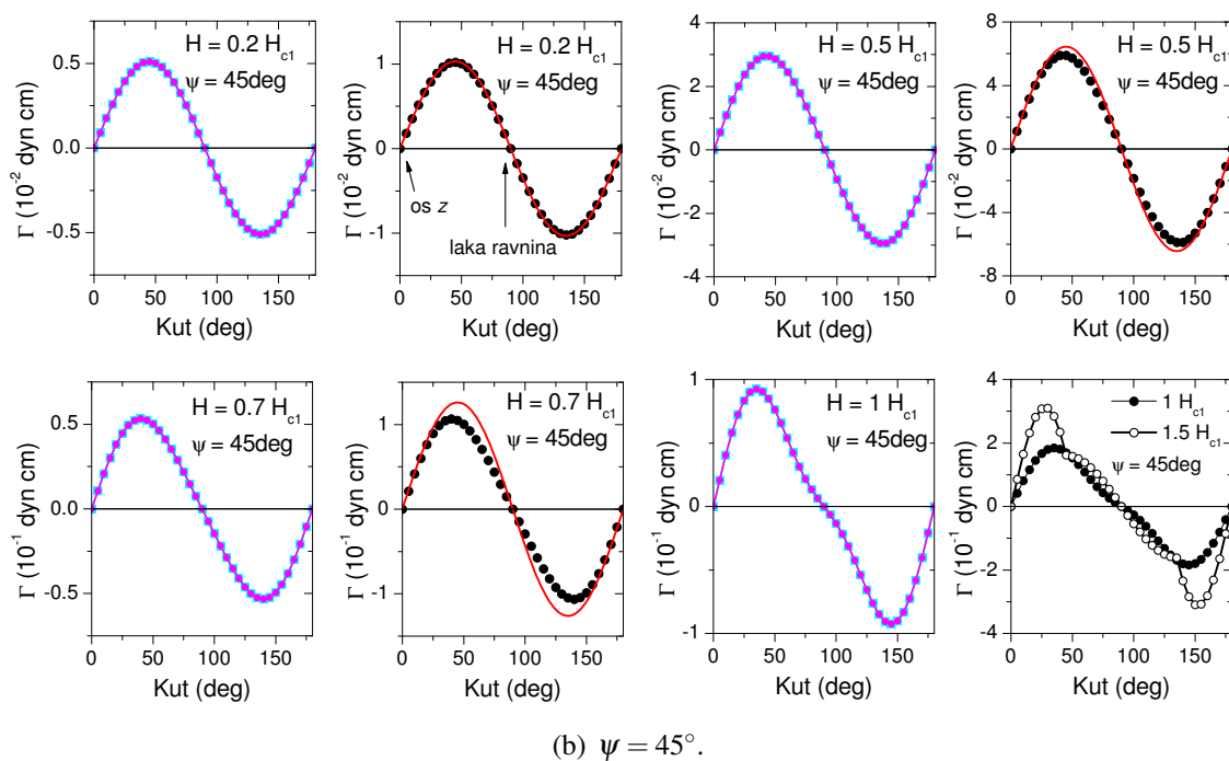
Slika 5.14 – Kutna ovisnost momenta sile u antiferomagneta sa simetrijom lake ravnine u ravnini koja sadrži tvrdu os. Kut \psi predstavlja kut koji projekcija polja zatvara sa smjerom lake osi. Smjer osi z na kutu 0^\circ odn. 180^\circ je smjer najvećeg iznosa magnetokristalne energije. Plave i ružičaste točke predstavljaju momente sile u pojedinim domenama, a crne ukupni moment sile. Crvene krivulje predstavljaju pravilne sinusoide dobivene množenjem sinusoide na 1\text{kOe} s H^2/1000^2 . m = 0.00128\text{ g} , M_{mol} = 545\text{ g/mol} , a konstante anizotropije i iznosi pojedinih susceptibilnosti imaju vrijednosti kao na slici 5.11.
