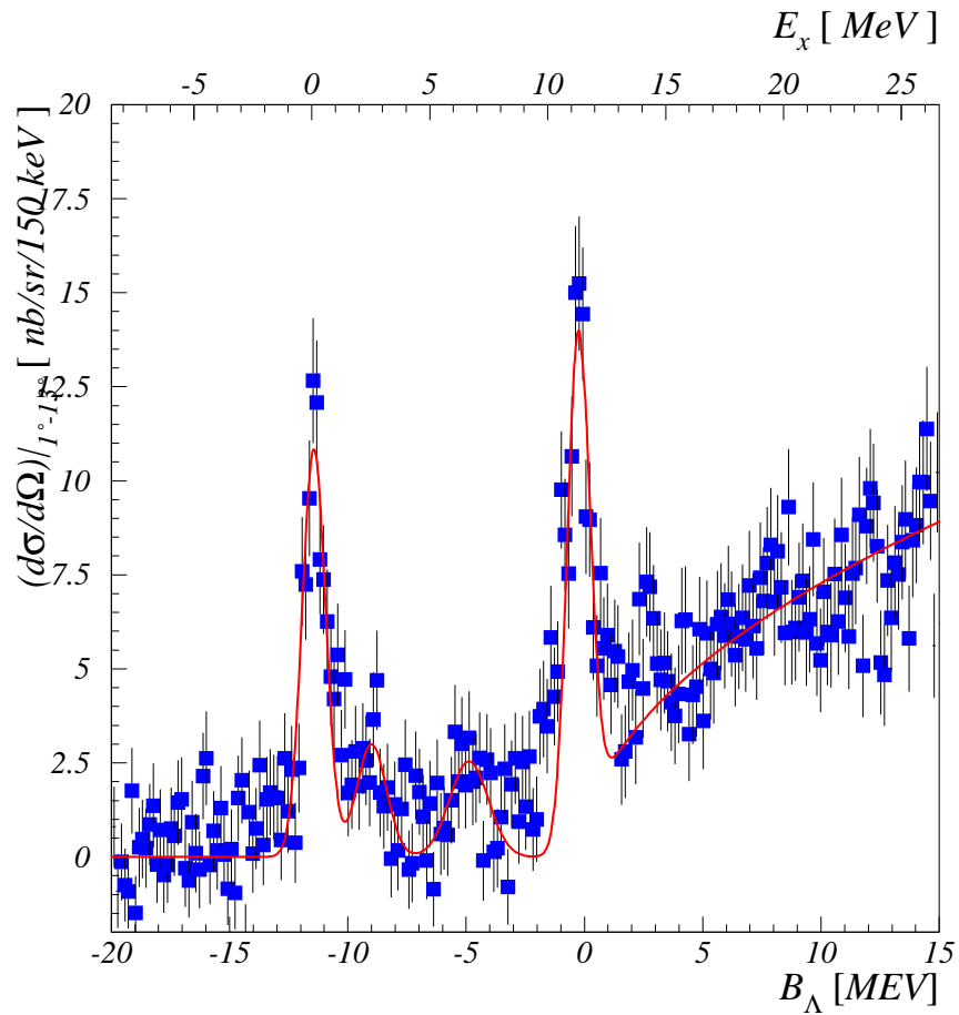
(c) Prezentirana studija, JLab Hall C : E01-011
