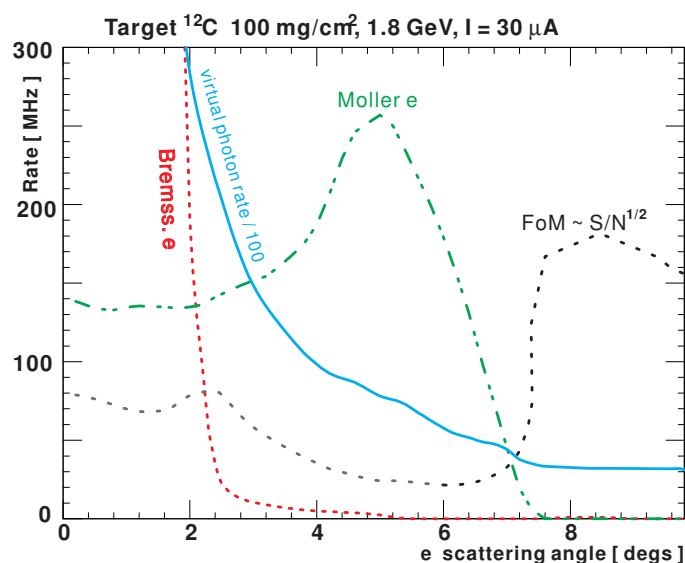
SLIKA 2.6: KUTNA OVISNOST PRODUKCIJE ELEKTRONA ZAKOČNIM ZRAČENJEM, MOLLER RASPRŠENIH ELEKTRONA I TOKA VIRTUALNIH FOTONA ZA 12 C METU GUSTOĆE 100 MG/CM 2 I STRUJE ELEKTRONSKOG SNOPA OD I=30μA. FIGURE OF MERIT (FoM) DEFINIRAN JE KAO FoM = S/N^{1/2} , S- TOK VIRTUALNIH FOTONA; N - SUMA ELEKTRONA PRODUCIRANIH ZAKOČNIM ZRAČENJEM I MOLLER RASPRČENIH ELEKTRONA. TOK VIRTUALNIH FOTONA I FoM SU SKALIRANI RADI GRAFIČKOG PRIKAZA. [13].
