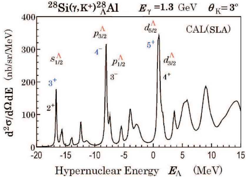
SLIKA 5.7: TEORIJSKI PREDVIĐEN SPEKTAR ZA ^{28}\text{Si}(\gamma, K^+)\Lambda^{28}\text{Al} REAKCIJU. RAČUN JE RAĐEN S E_\gamma = 1.3 \text{ GeV} I \theta_{K^+}^{LAB} = 3^\circ U SLA IZOBARNOM MODELU [31] [33].
