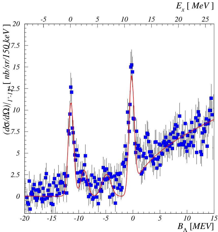
(a) KEK-E369: (\pi^+, K^+) reakcija [15] (b) INFN-DAΦNE: (K^-, \pi^-) reakcija [22]
