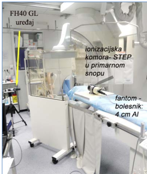
Slika 9.1. Al debljine 4 cm – rendgenskom uređaju pripadajući originalni fantom trupa bolesnika – sekundarni izvor raspršenog zračenja STEP ionizacijska komora volumena 1 l – priznati instrument za mjerenja u pulsним poljima i FH 40GL mjerne sonde.
