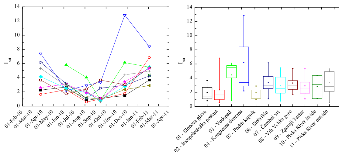
Figure 7.21 I_{\text{sat}} values calculated for drip waters and in Pivka River, in the sampling period Slika 7.21 Vrijednosti I_{\text{sat}} računate za prokapnicu i Pivku tijekom perioda uzorkovanja.
