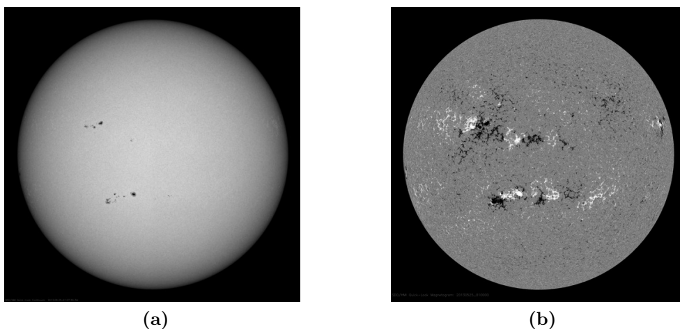
Slika 1.1.: Usporedba Sunca u (a) vidljivoj svjetlosti i (b) magnetogramu 25. svibnja 2013. Bijela područja na magnetogramu označavaju sjeverni magnetski polaritet, a crna područja južni polaritet. Ljubaznošću NASA/SDO.
