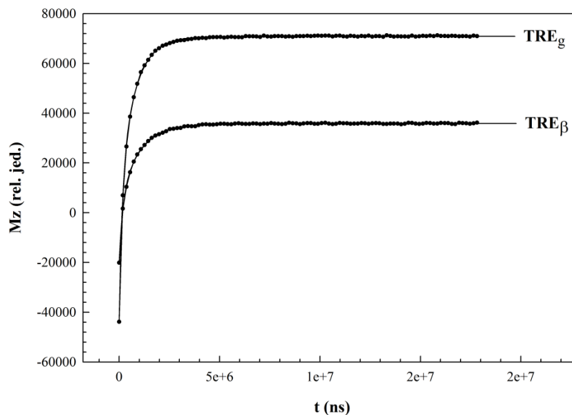
Slika 4.3: Magnetizacijske krivulje na 80 K za uzorke trehaloze u polikristalnom ( TRE_{\beta} ) i staklastom ( TRE_g ) stanju. Pune linije predstavljaju prilagodbu eksperimentalnih podataka ( \bullet ) na dvoeksponencijalnu funkciju.
