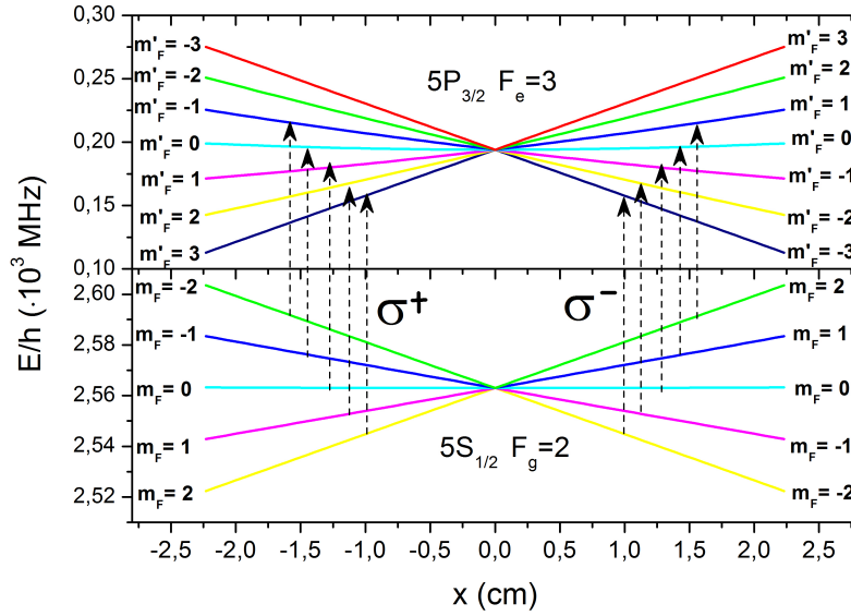
Slika 2.12: Cijepanje magnetskih podnivoa u ovisnosti o pomaku od centra stupice. Strelicama su označeni dozvoljeni \sigma^+ i \sigma^- prijelazi.
