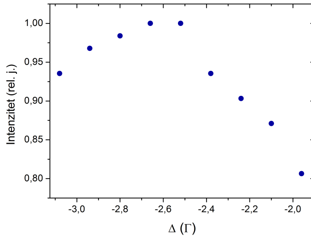
Slika 4.13: Intenzitet fluorescencije hladnih atoma u ovisnosti o frekventnom pomaku lasera za hlađenje od rezonancije uz b = 13 Gauss/cm.
