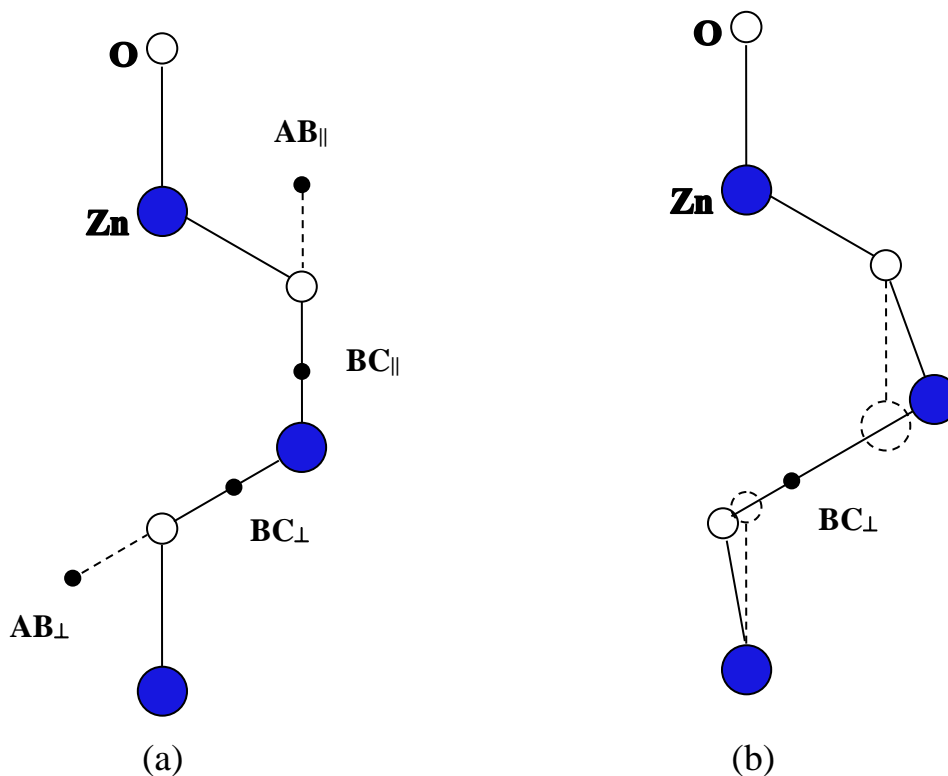
Slika 5.48: (a) Shematski prikaz položaja intersticijskih H atoma u (11-20) ravnini wurzitnog ZnO. (b) Atomski položaji intersticijskog H atoma i atoma ZnO matrice nakon relaksacije za BC_{\perp} konfiguraciju. Položaji atoma nerelaksirane rešetke su označeni isprekidanim crtama. Na slici plavi kružići označavaju Zn atome, dok su O atomi prikazani bijelim kružićima, a H atomi malim crni kružićima.
