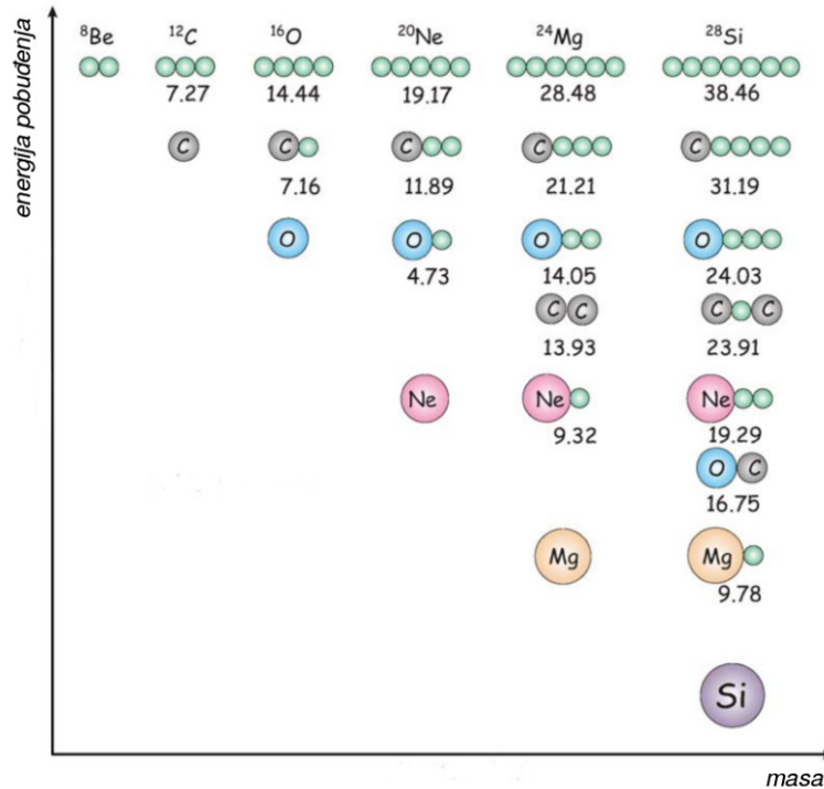
Slika 2.3: Ikedin dijagram \alpha -konjugiranih jezgara. Klasterne strukture nalaze se u blizini pragova za raspad jezgre na pojedine klasterne. Energije potrebne za taj raspad (u MeV-ima) naznačene su na slici iznad shematskog prikaza klasterne stanja jezgara [26].
