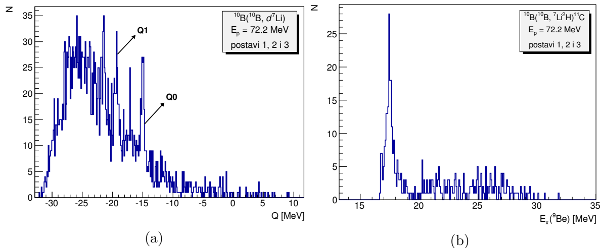
Slika 5.44: (a) Q-spektar reakcije u kojoj detektiramo ^7\text{Li} i ^2\text{H} u koincidenciji, za mjerenja na 72.2 MeV, s uključenim svim postavama i kombinacijama detektora; (b) Energija pobuđenja jezgre ^9\text{Be} iz koincidencija ^7\text{Li} i ^2\text{H} s uključenim svim postavama i oba vrha Q-spektru, Q0 i Q1.
