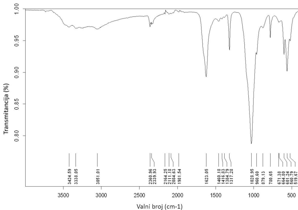
Slika 20. FT-IR spekter uzorka OS4b. (ATR), \tilde{\nu}_{\max}/\text{cm}^{-1} : 3333 (O-H istezanje), 1623 (C=O istezanje), 1317 (C-O istezanje), 1028 ( \text{PO}_4^{3-} istezanje), 519 (O-C-O istezanje).
