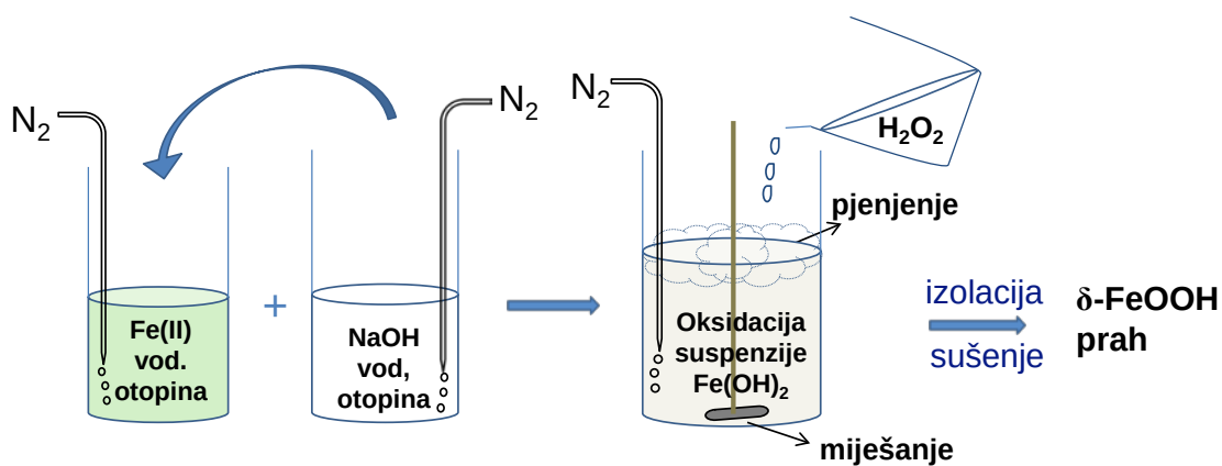
Slika 15. Shematski prikaz sinteze nanočestica \delta -FeOOH klasičnim postupkom taloženja Fe(II) iona s vodenom otopinom NaOH u inertoj atmosferi, a nanočestice \delta -FeOOH nastaju bržom oksidacijom željezovog(II) hidroksida uslijed dodavanja vodikovog peroksida ( \text{H}_2\text{O}_2 ) (Gotić i sur., 1994).
