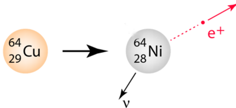
Slika 5.8: Prikaz \beta^+ raspada.
