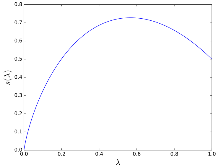
Slika 3.3: Specifična mikrokanonska entropija konfiguracijskog modela za k -regularne grafove u slici bridovi-ka0-čestice
