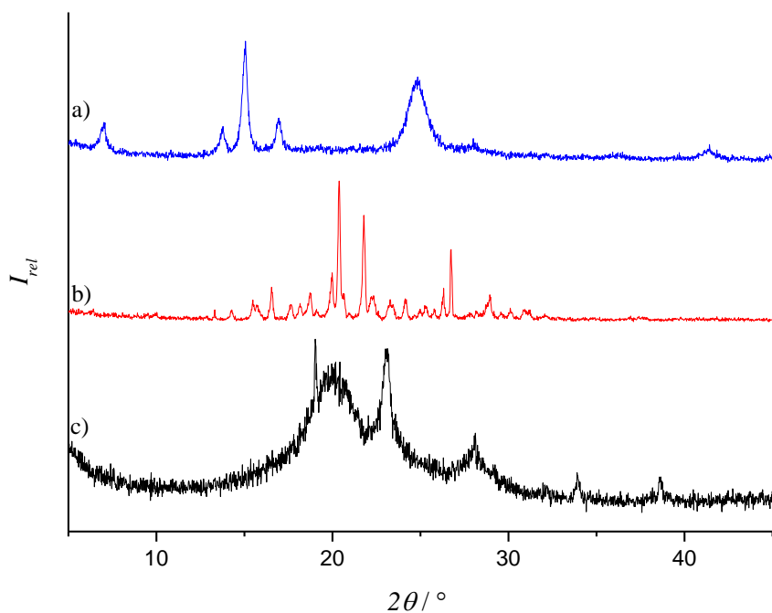
Slika 26. Usporedba difraktograma praškastih uzoraka a) reaktanta 1 , b) reaktanta 2a te c) azo spoja 2 .
