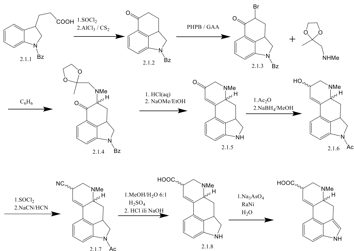
Shema 1. Sintaza lizerginske kiseline prema Kornfeldu, Woodwardu i suradnicima
