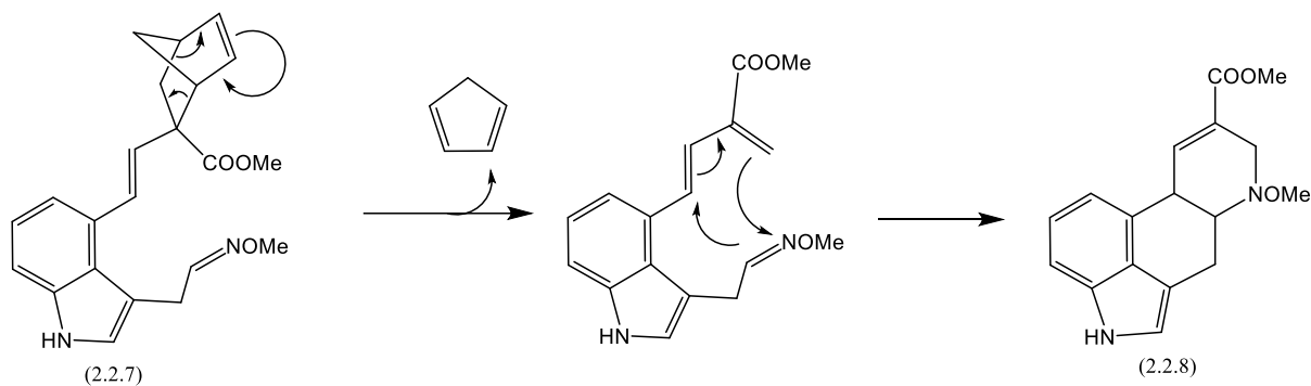
Shema 3. Mehanizmi retro-Diels-Alderove reakcije i intramolekuske Diels-Alderove reakcije kojima iz spoja 2.2.7 nastaje spoj 2.2.8
