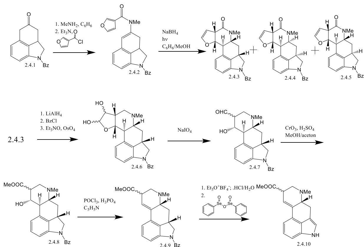
Shema 6. Sinteza lizerginske kiseline fotociklizacijom enamida prema Ninomiyyi i suradnicima
