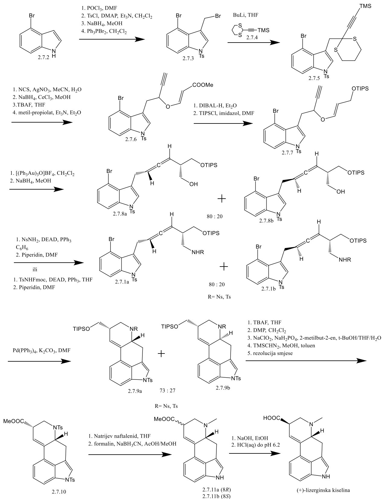
Shema 14. Sinteza lizerginske kiseline domino ciklizacijom alena prema Fujiju, Ohnou i suradnicima
