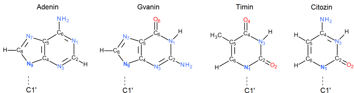
Slika 1.3 Dušične baze.
