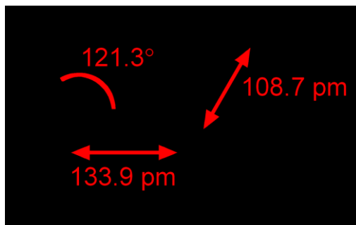
Slika 2. Struktura molekule etena C_2H_4 . 8
