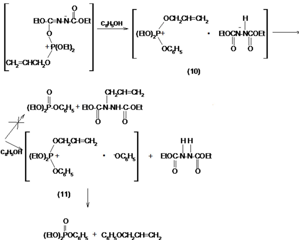
Slika 19: fosforilacija fenola uz dobivanje dietil-fenil fosfata, dietilhidrazodikarboksilata i alil-fenil-etera
