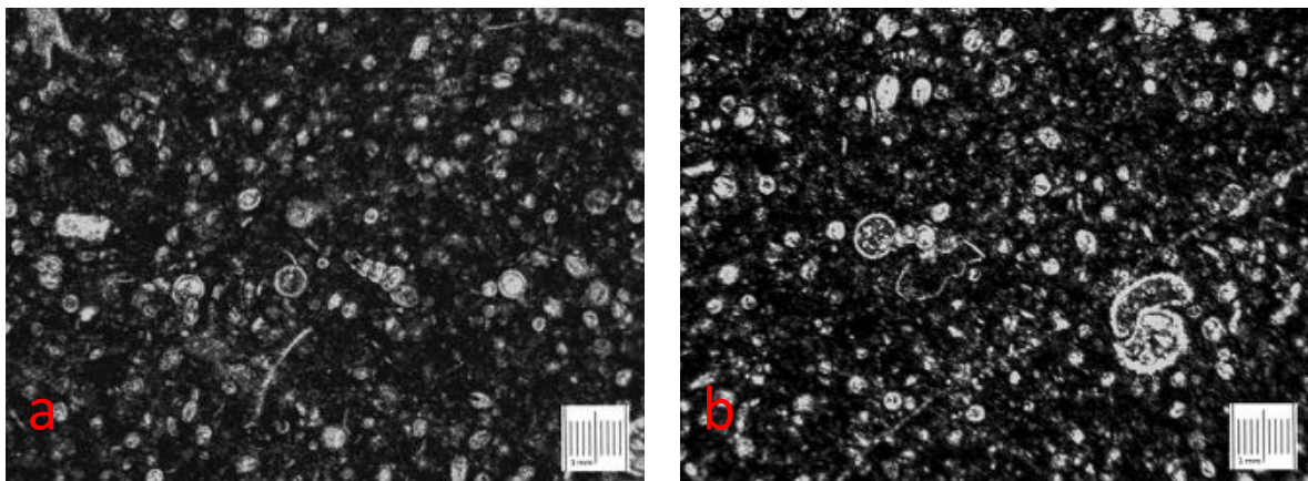
Slika 19) Biomikrit s kalcisferama i pitonelama ( a, b uzorak T-9, točka TV7).
