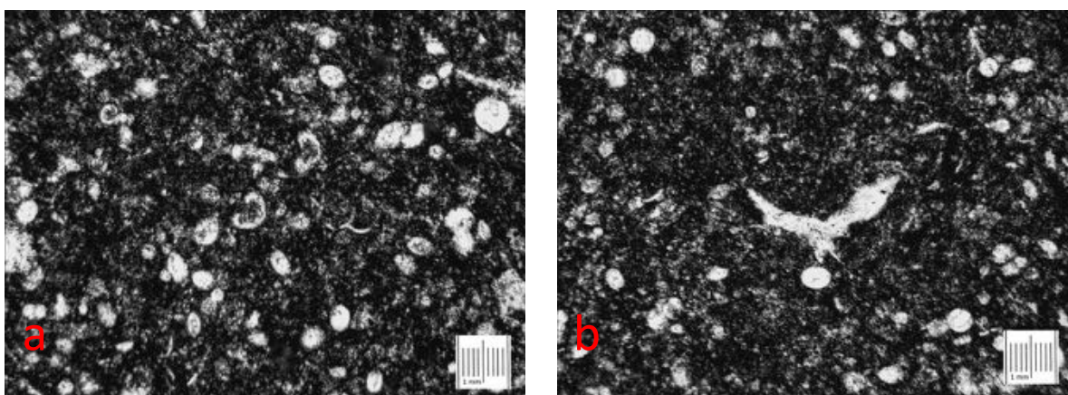
Slika 20) Biomikrit s kalcisferama i pitonelama, fragmentima krinoida i rijetkim planktonskim foraminiferama ( a, b uzorak/točka 1168).
