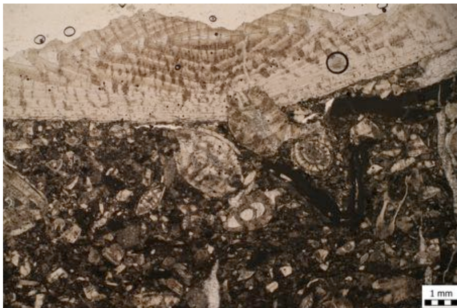
Slika 30) Numuliti. Uzorak T-16, točka TV13.
