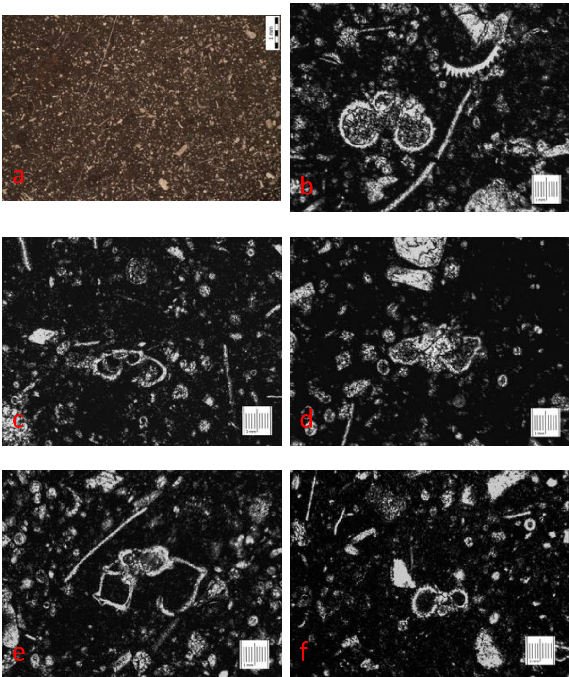
Slika 13) Biomikrit s planktonskim foraminiferama (uzorak T-4 a–f , točka TV2).
