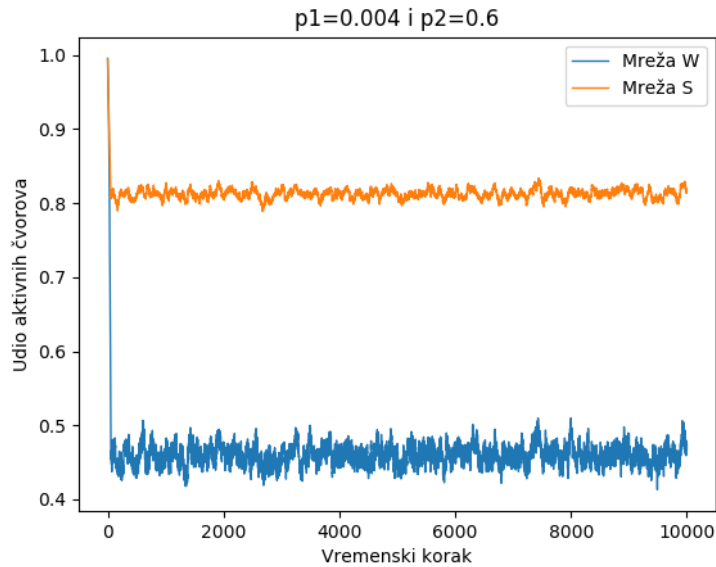
Slika 6.1: Simulacija udjela aktivnih čvorova u vremenu za vjerojatnosti neuspjeha p_1 = 0.004 i p_2 = 0.6 . Mreže S i W su u početnom trenutku stavljene u potpuno aktivno stanje. Pragovi su stavljene na T_s = 0.3 i T_w = 0.7 . Otpornija mreža S je označena narančastom bojom, dok je mreža W označena plavom bojom
