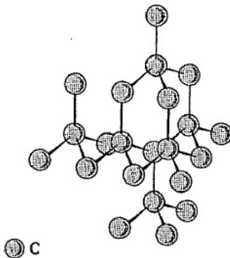
Slika 2. Struktura dijamanta
