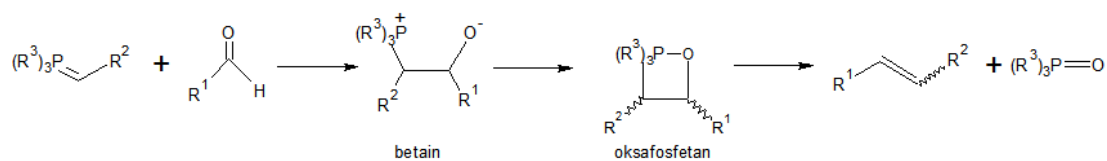
Slika 11. Betain mehanizam. 3
