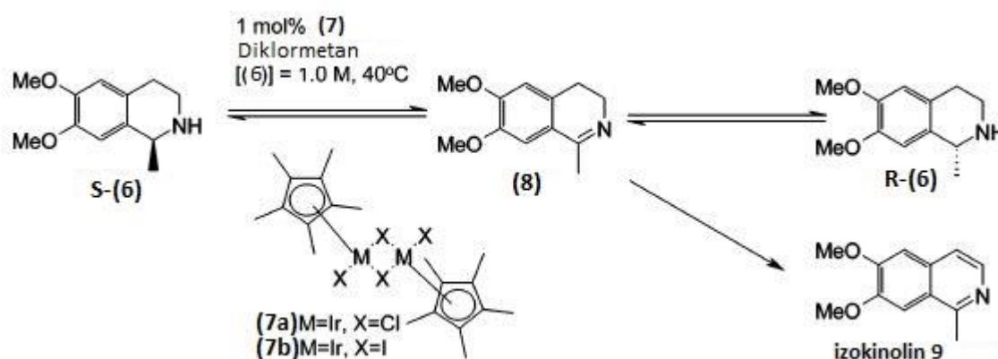
Shema 9. Dehidrogenacija i racemizacija (1S)-6,7-dimetoksi-1-metil-1,2,3,4-tetrahidroizokinolina uz korištenje [\text{IrX}_2\text{Cp}^*]_2 katalizatorskog kompleksa 16
