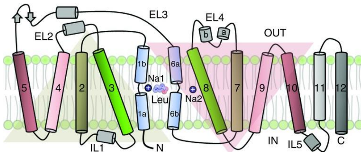
Slika 4. Strukturalna organizacija bakterijskog LeuT transportera (homologa SERT-a), opisana kao pseudosimetrično uređenje 12 heliksa od kojih je sastavljen 7
