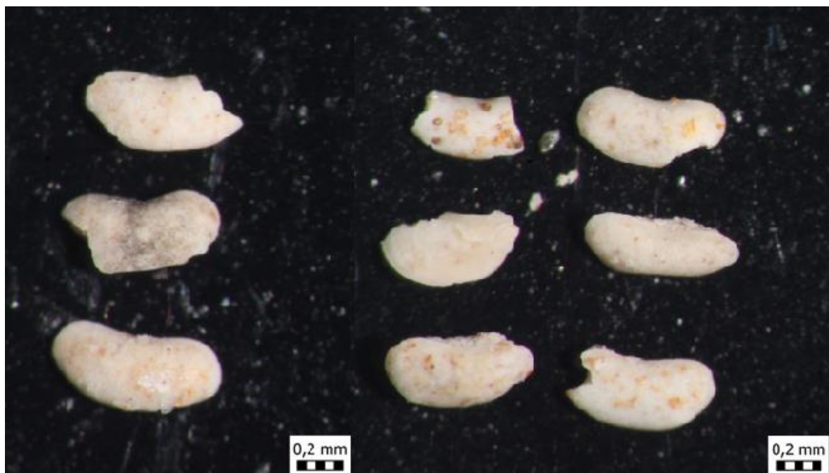
Slika 12. Ljuštore ostrakoda
