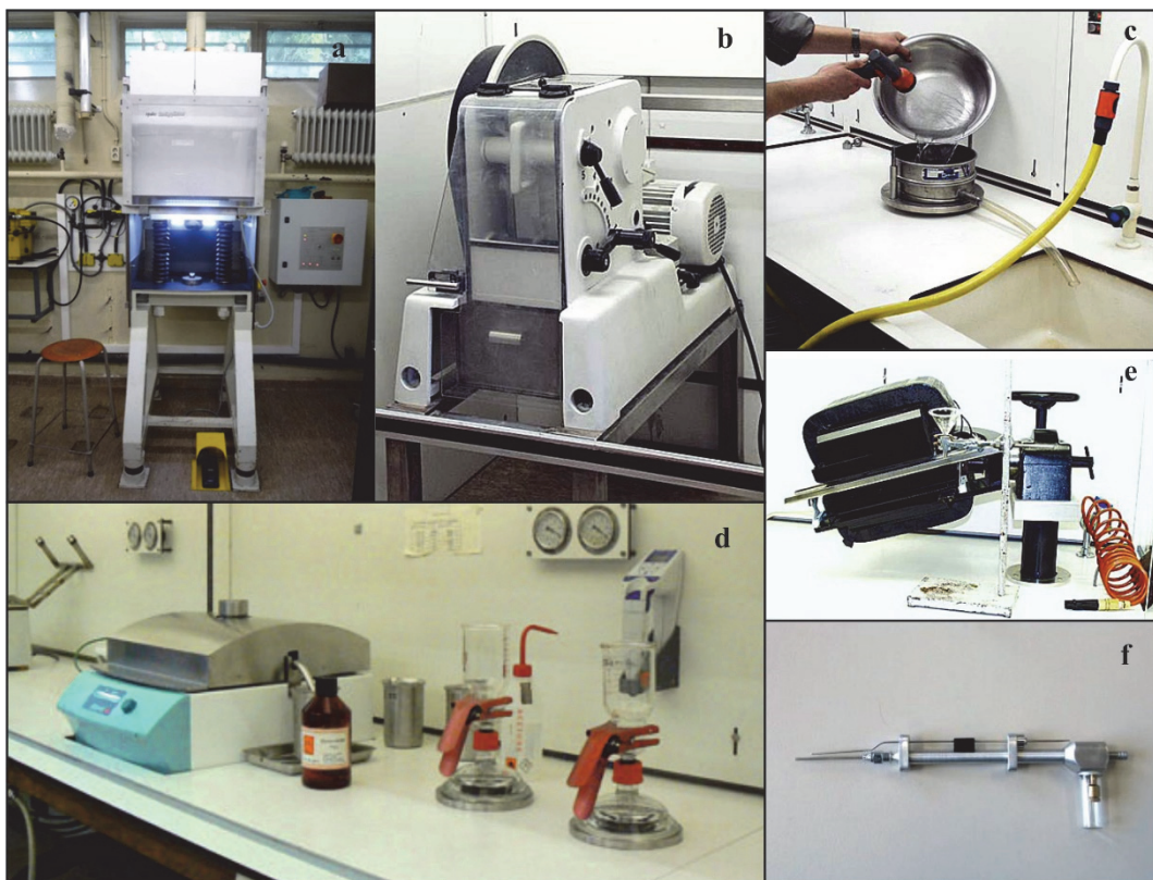
Slika 3.1. Instrumenti korišteni za separaciju minerala. a) cjepač stijena ( rock splitter ), b) drobilica stijena, c) Sito za sijanje, d) Frantzov magnetni separator, e) Centrifuga i instrumentarij za separaciju teškim tekućinama, f) Alat za izdvajanje. Slike su preuzete s web izvora: http://www.falw.vu.nl/nl/onderzoek/laboratoria/labs-aardwetenschap/mineral-separation-laboratory/index.aspx .
