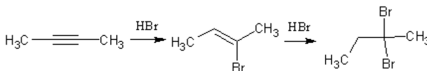
Slika 4: Adicija bromovodika na but-2-in
