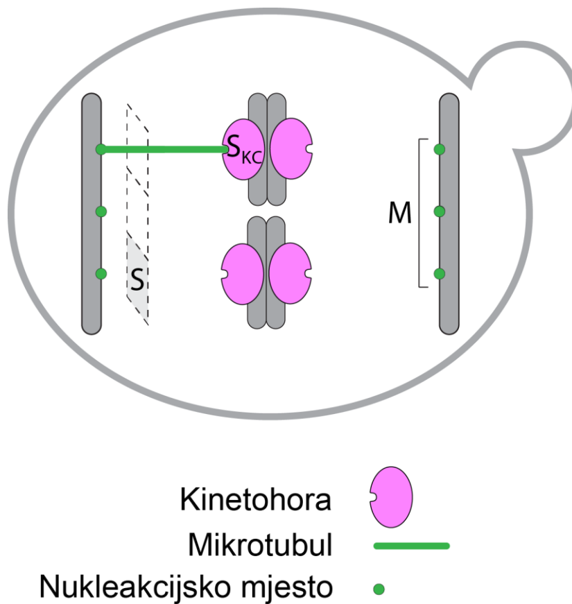
Slika 5. Shema dijelova stanice najvažnijih za model. Površina S označava površinu jednog nukleacijskog mjesta na spindle pole body -u (dugački sivi štap na slici), dok površina S_{KC} označava površinu kinetohore na kromosomu (kratki sivi štap). Broj M je broj nukleacijskih mjesta iz kojih nukleiraju mikrotubuli.
