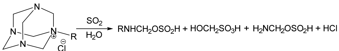
Shema 4. Prikaz dobivanja alkil aminometil sulfita (RNHCH 2 OSO 2 H).
