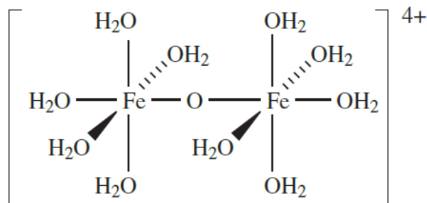
Slika 4. [(\text{H}_2\text{O})_5\text{FeOFe}(\text{OH})_5]^{4+} kompleksni ion nastao uslijed hidrolize [\text{Fe}(\text{OH})_6]^{3+} iona. 4
