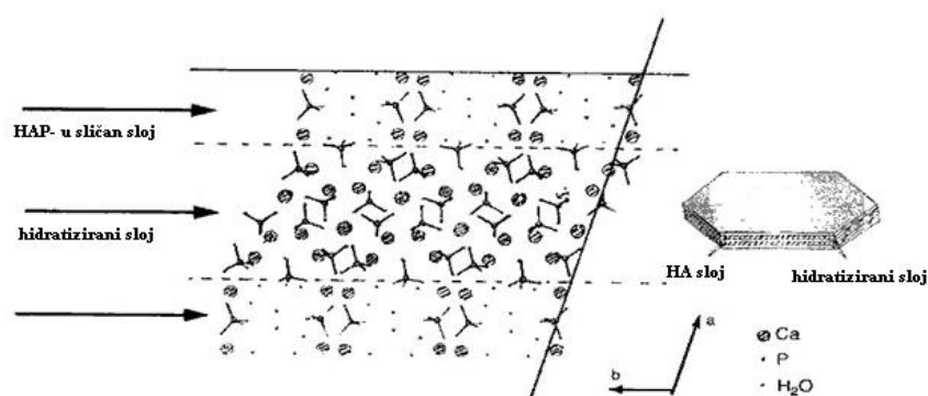
Slika 7. Struktura i tipična morfologija oktakalcijeveg fosfata. Konstruirano prema referenci [1].
