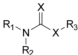
Slika 8. Općenita struktura biološki aktivnih karbamata
