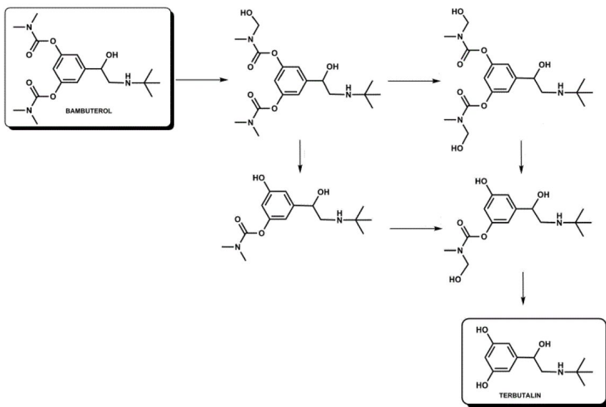
Shema 3. Transformacija dikarbamatnog prolijeaka bambuterola u antiasmatik terbutalin uz BChE
