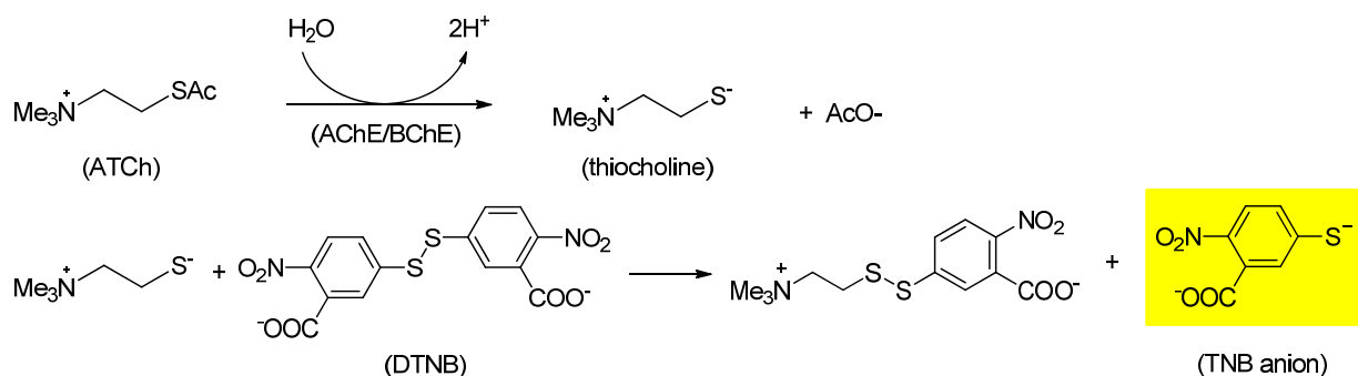
Shema 8. Ellmanova metoda za određivanje aktivnosti kolinesteraza. Tiokolinatni anion koji nastaje kao produkt enzimske reakcije reagira s DTNB čime nastaje žuto obojeni TNB anion
