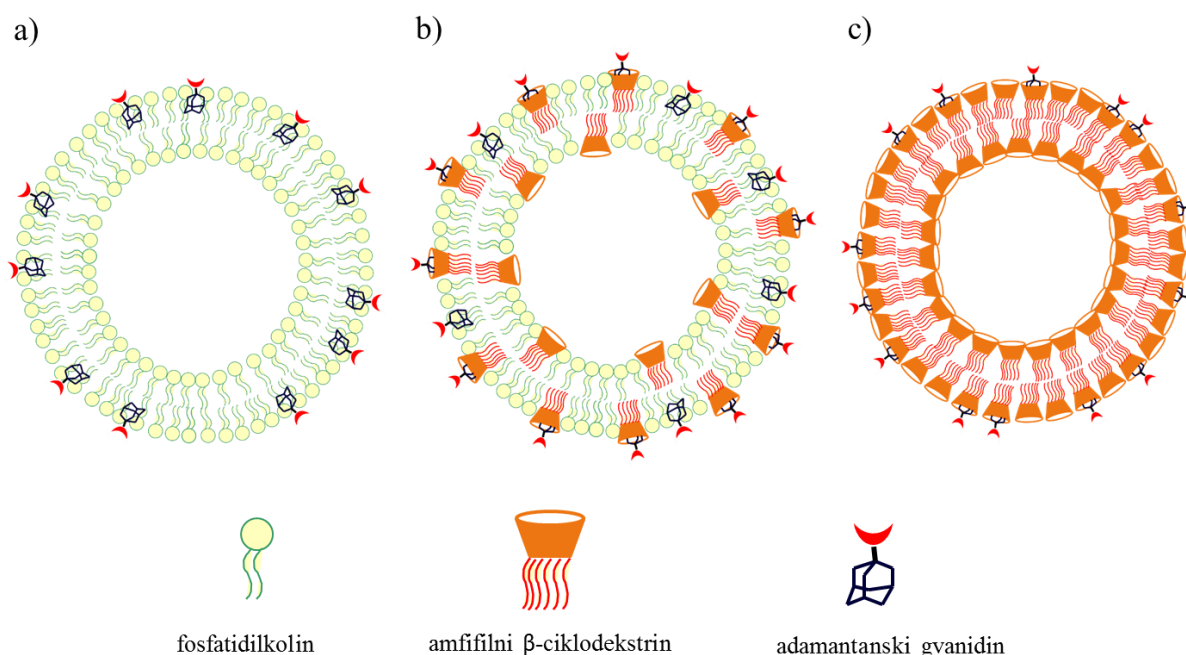
Slika 16. Shematski prikaz pripremljenih funkcionalnih supramolekulskih sustava temeljenih na kompleksima liposoma i amfifilnog ciklodekstrina s adamantanskim gvanidinima. a) PC liposomi s AG, b) PC : EO-CE-SR liposomi s AG, c) EO-CE-SR vezikule s AG
