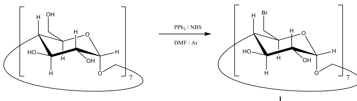
Shema 3. Shematski prikaz priprave spoja heptakis-(6-deoksi-6-bromid)-β-ciklodekstrina 1
