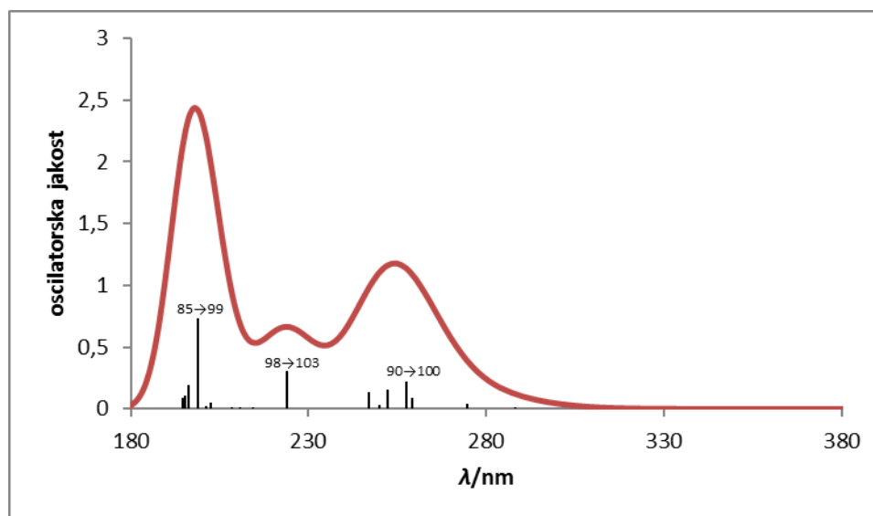
Slika 19. Grafički prikaz simuliranog UV/vis spektra molekule 3 u acetonitrilu. Pobudne energije i oscilatorske jakosti izračunane su TD-CAM-B3LYP metodom.
