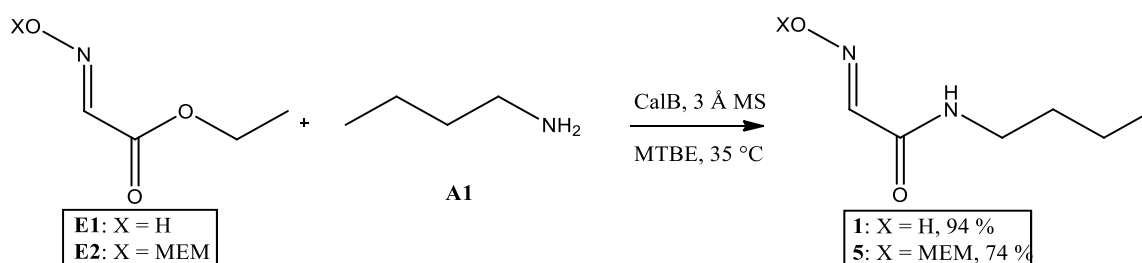
Slika 42. Sinteza N -butil-2-(hidroksiimino)acetamida 1 i N -butil-2,5,7-trioksa-8-azadec-8-en-10-ovata 5 metodom enzimske katalize
