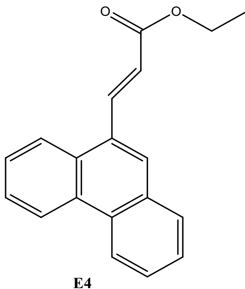
Slika 26. Strukturna formula estera etil-( E )-3-(fenantr-9-il)-2-propenoata E4
