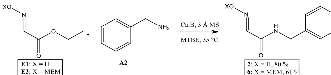
Slika 43. Sinteza N -benzil-2-(hidroksiimino)acetamida 2 i N -benzil-2,5,7-trioksa-8-azadec-8-en-10-ovata 6 metodom enzimske katalize
