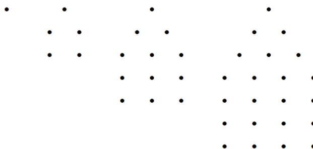
Slika 10: Peterokutni brojevi
