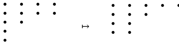
Slika 6: Konjugacija particije (4, 4, 2, 1, 1)
