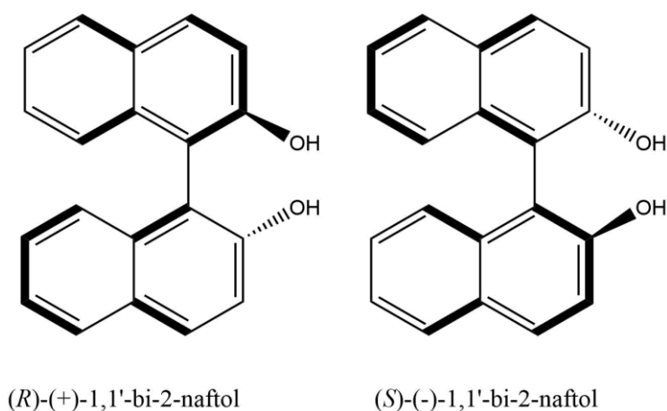
Slika 2. Enantiomeri 1,1'-bi-2-naftola
