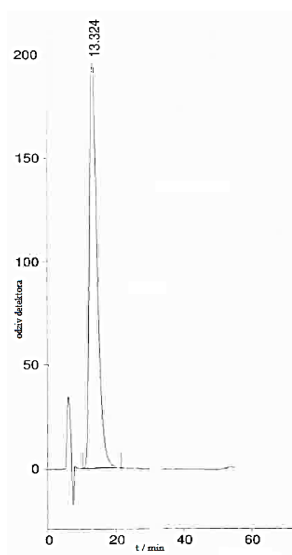
Slika 17. Kromatogram ( S )-(-)-2,2'-bis(difenilfosfino)-1,1'-binaftalena
