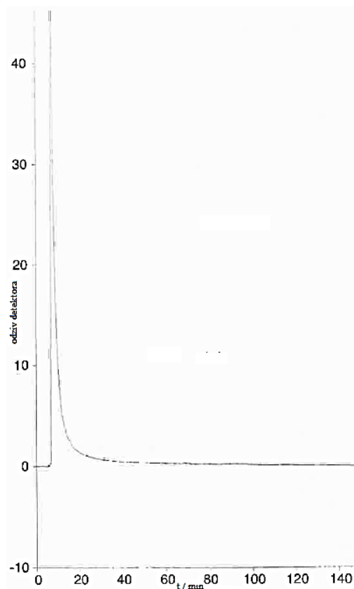
Slika 16. Kromatogram ( R )-(-)-1,1'-binaftil-2,2'-diilhidrogenfostata
